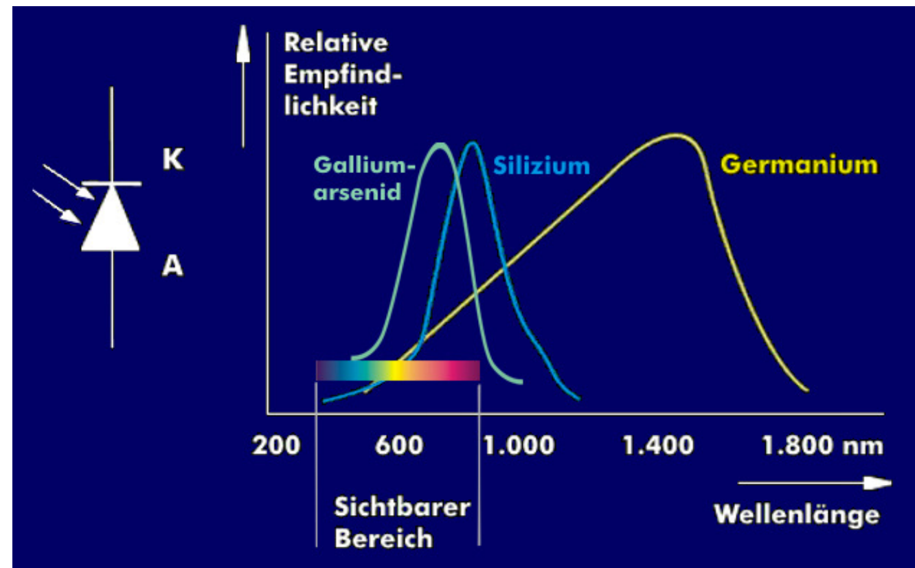
Kennlinien von Fotodioden aus Silizium und Germanium
