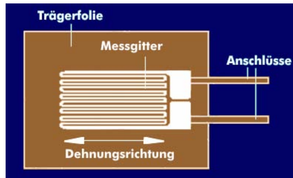
Aufbau eines Dehnungsmessstreifens
