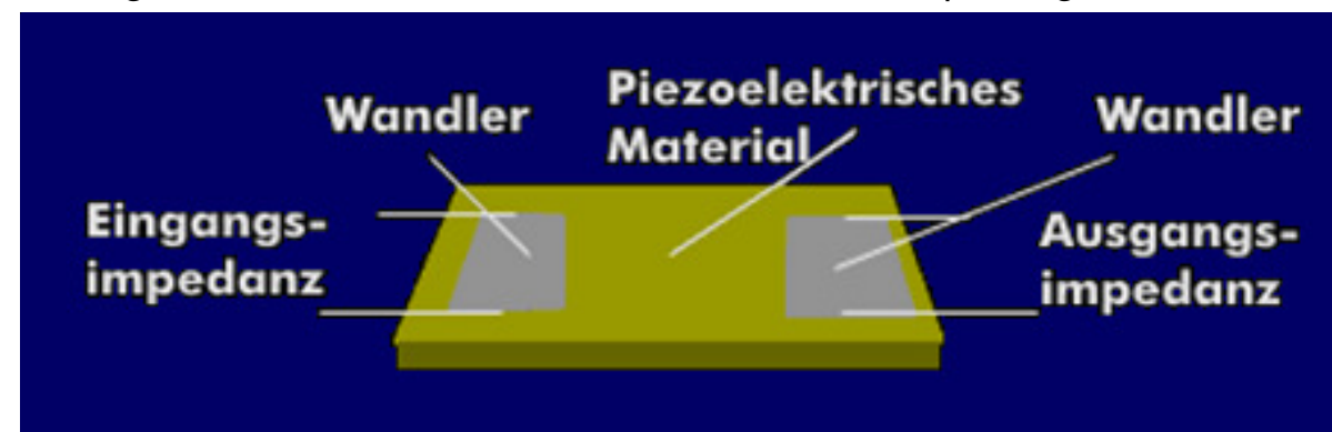
Aufbau eines Oberflächenwellenfilters
