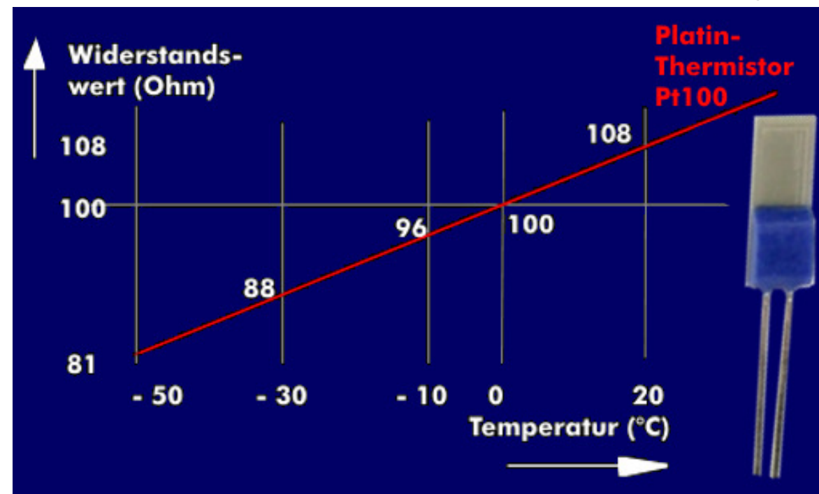
Widerstandskennlinie und Pt100-Thermistor in Dünnschichttechnik
