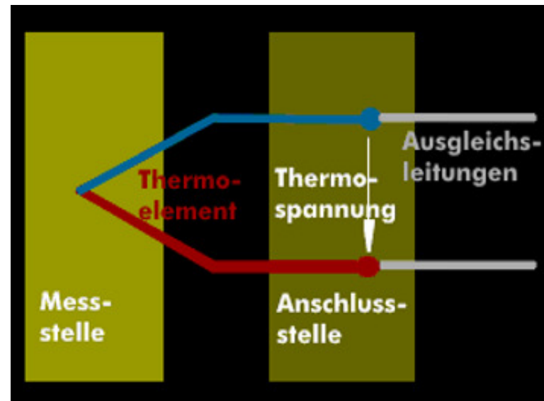
Prinzipieller Aufbau eines Thermoelements
