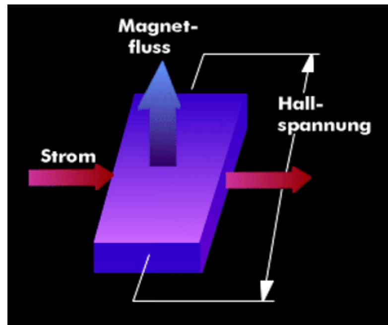
Generierung der Hallspannung durch Magnetfluss und Stromfluss
