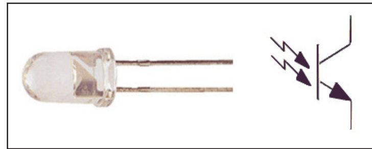
Fototransistor und Schaltzeichen, Foto: Kingbright
