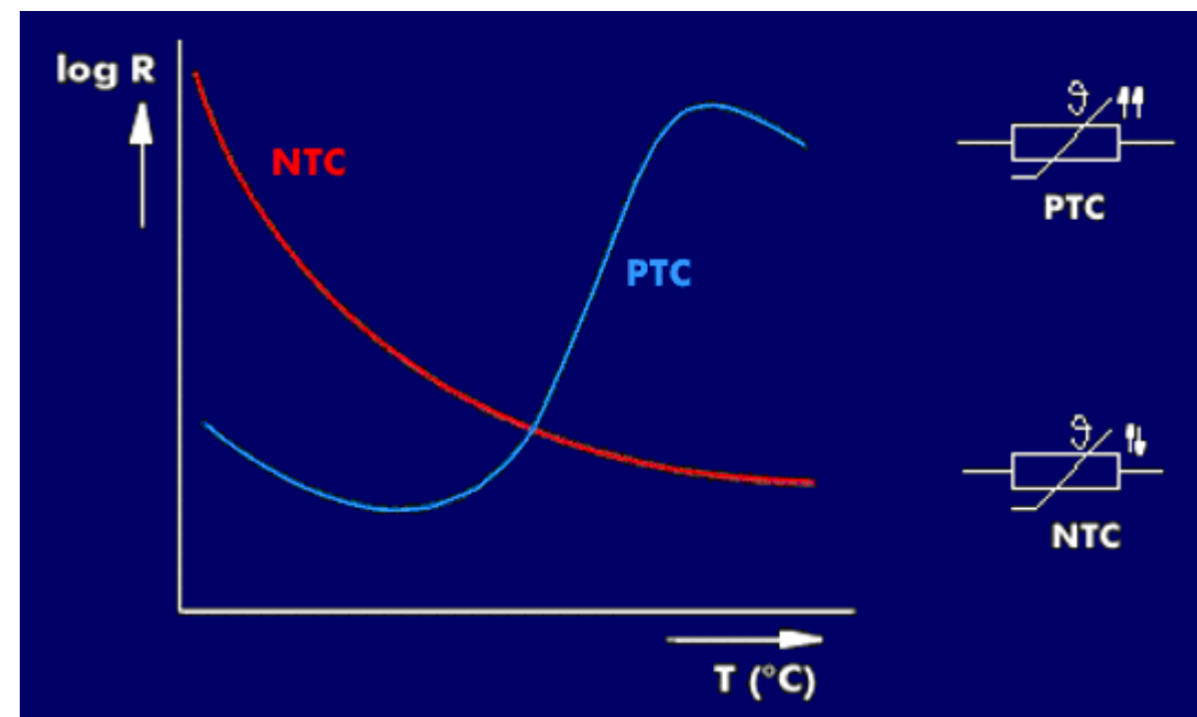
Kennlinien von NTC- und PTC-Thermistoren
