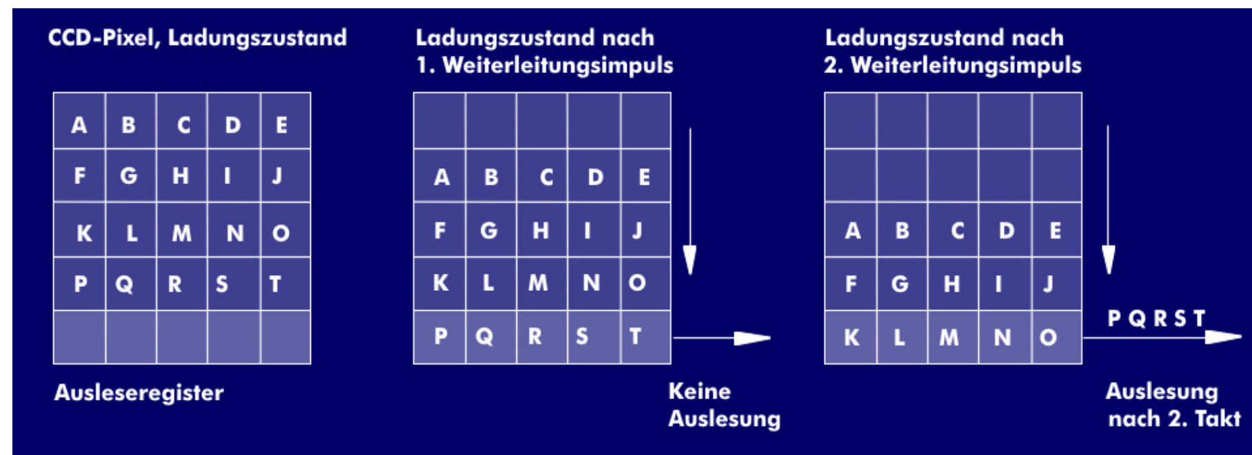
In CCD-Sensoren angewandtes Eimerkettenprinzip
